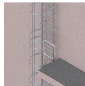
Selbstschließende Tür zu Steigleiter für Seitenausstieg
