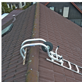
First-Überwurfbügel
