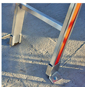
Paar Bodenwinkel für Sprossenleitern für Profil 70
