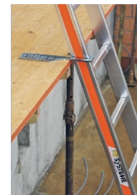
Stk. Sicherungshaken für Anstellleiter
